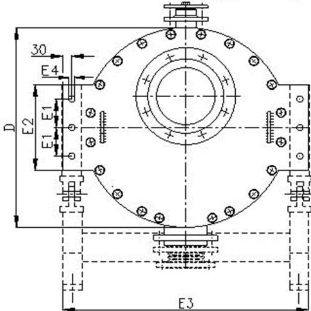
Ansicht C
