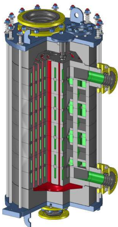
GMP Graphit-Ringnutkondensator im Schnitt
