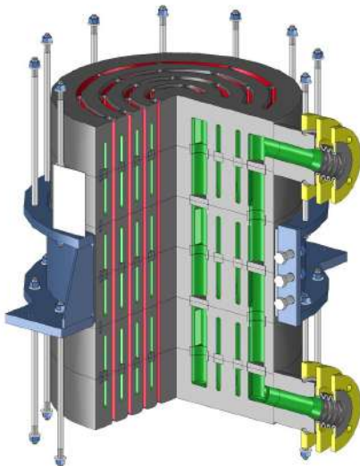
Graphit-Ringnutwärmeübertrager zum Direkteinbau in Kolonnen im Schnitt
