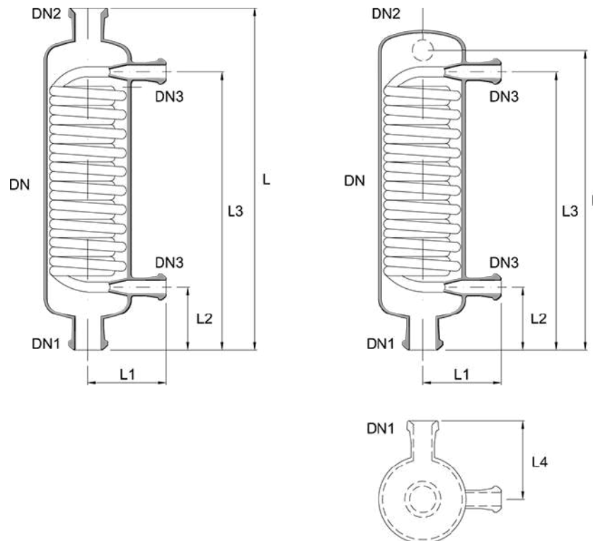
Nachkondensator, vertikal, HGV...-K
