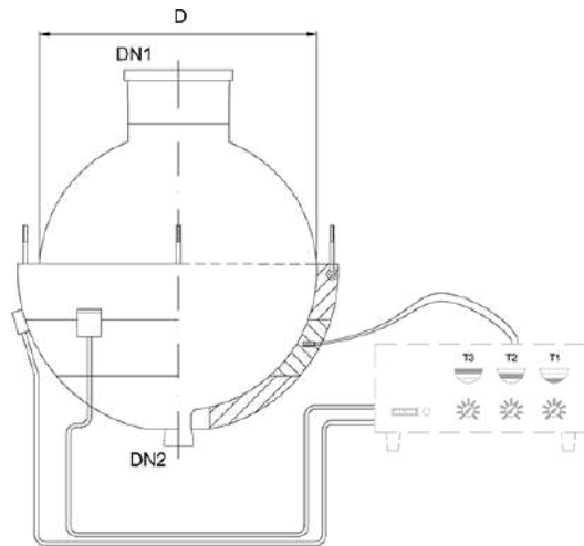
Heizpilz HHC für Kugelgefäße
