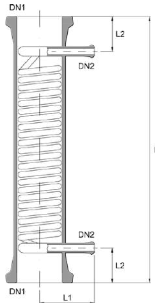
Schlangen-Wärmeübertrager HC...-K
