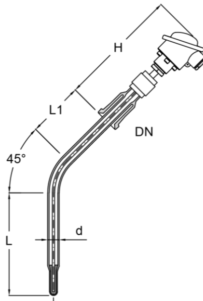
Widerstandsthermometer, abgewinkelt MTT45/...-K
