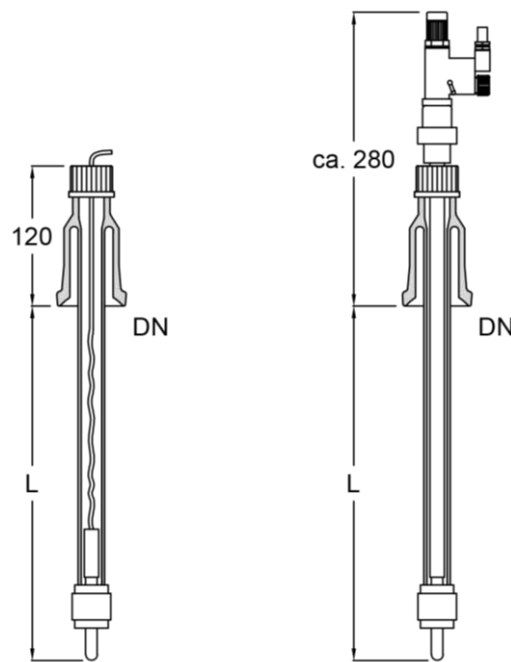
pH-Messung MpHT / MpHV ..., System „Standard“ MpHT..., System „PFAUDLER“
