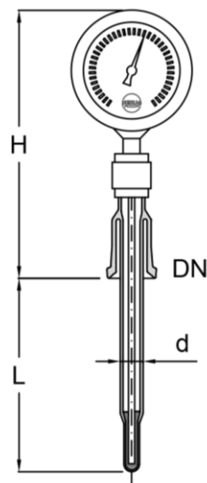
Bimetallthermometer, gerade MTI...-K
