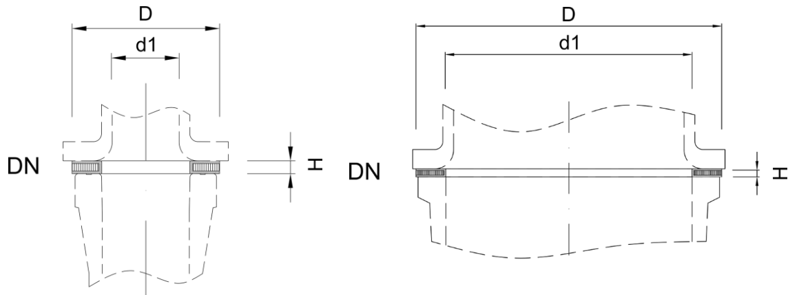
Flachdichtung für mehrfaches Öffnen und Schließen, Typ CGP... für Glasanschluss bis DN 150
