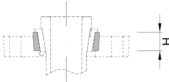
Übergangseinlage, Typ CIPE... für Sicherheitsplanflansch (PF) auf Bundflansch (KF) bzw. EN 1092-1
