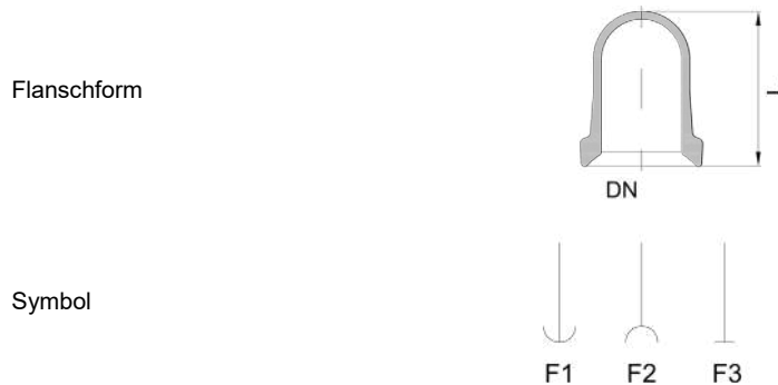
Blindflansche PC...-F1...F3
